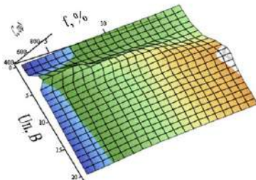
Рис. 1. Зависимость емкости C = f(\varphi; U_{\Pi}) при d = 0,1 мм и t = 45^{\circ}\text{C}
