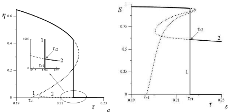
Рис. Температурные зависимости параметра порядка (а) ЖК \eta и (б) магнито-дипольных УНТ S для \xi = 10^4 , \zeta = 10^4 , \omega = 10 , \omega_p = 0 , y_p = 0.02 , D_p = 2 \cdot 10^{-7} см и L_p = 2 \cdot 10^{-5} см. Кривая 1 – h = 0 ; кривая 2 – h = 10^{-4} . Пунктирная кривая отвечает метастабильным и неустойчивым состояниям.
