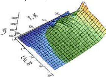
Рис. 3. Зависимости емкости C = f(T; U_{\Pi}) при d = 0,1 мм и \varphi = 8,3\%
