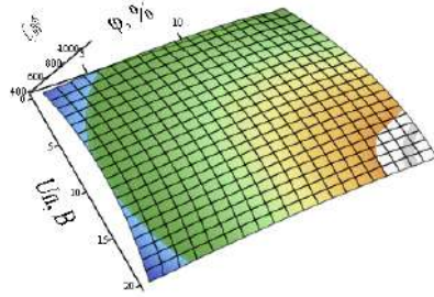
Рис. 6 – Зависимость емкости C = f(\varphi; U_{п}) при d = 0,1 мм и t = 65^\circ\text{C}
