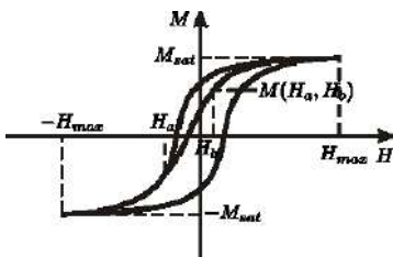
Рис. 4. Обратная кривая намагнитченности первого порядка
