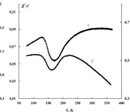
Рис. 3. Температурная зависимость магнитной восприимчивости образцов магнитного коллоида при воздействии внешнего постоянного магнитного поля H = 9,7 кА/м: 1 – образец №1, 2 – образец №2
