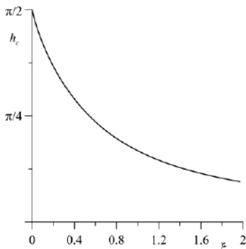
Рис. Зависимость критической напряженности магнитного поля h_c от параметра влияния поля \xi
