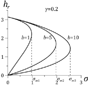
Рис. 2. Зависимость поля перехода h_r от энергии сцепления УНТ с ЖК-матрицей \sigma при различных значениях параметра b [ \sigma_{m1} = 0.972 , \sigma_{m2} = 1.973 , \sigma_{m3} = 2.554 ]
