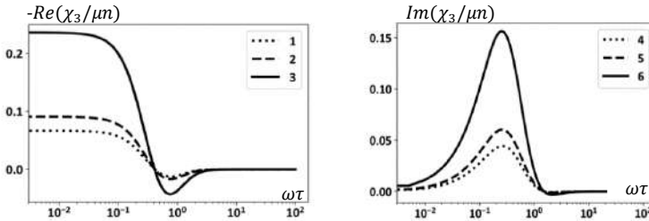
Рис.1. Графики мнимой и действительной частей кубической восприимчивости \chi_3 .
