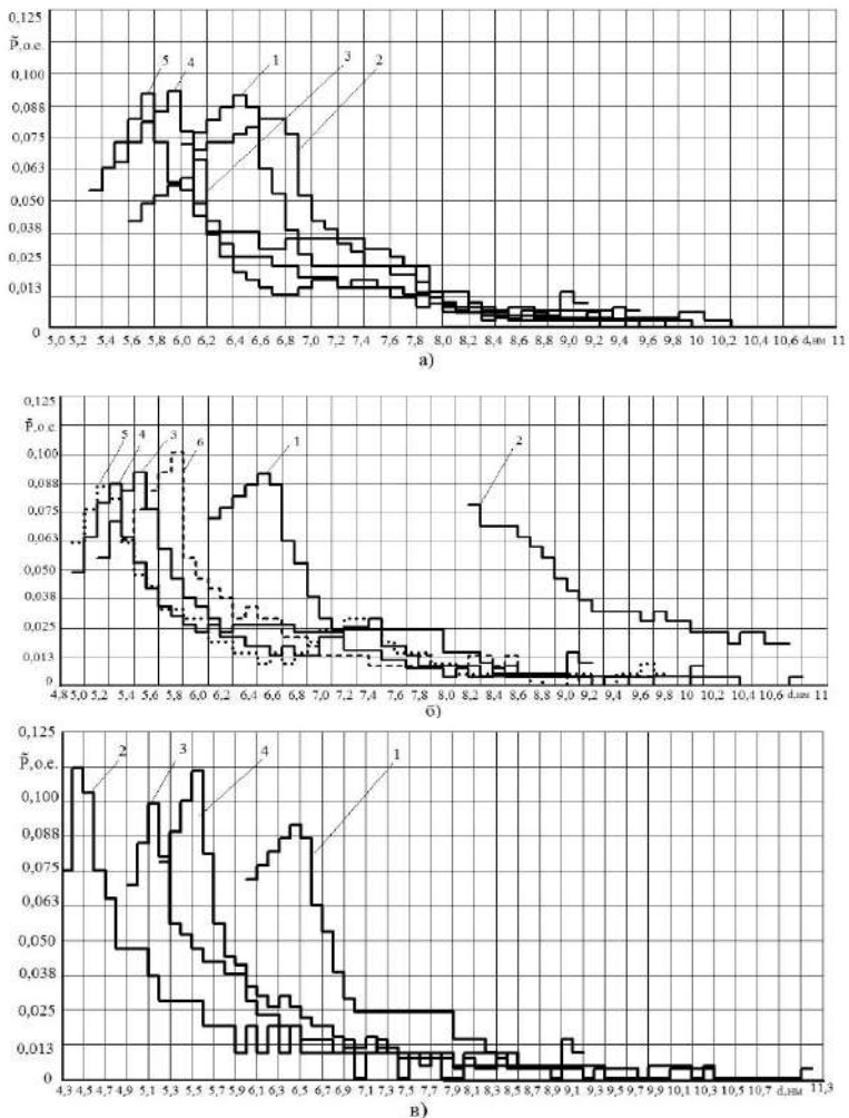
Рис. 5. Гистограмма распределения частиц МЖ после механического воздействия при частоте вращения активатора 500 об/мин. (а), 1000 об/мин. (б) и 2000 об/мин. при разном времени воздействия: 1 – исходная жидкость, 2 – 10 мин., 3 – 20 мин., 4 – 40 мин., 5 – 60 мин
