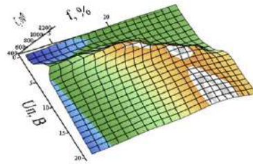
Рис. 2. Зависимость емкости C = f(\varphi; U_{\Pi}) при d = 0,1 мм и t = 85^{\circ}\text{C}
