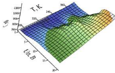
Рис. 4. Зависимости емкости C = f(T; U_{\Pi}) при d = 0,1 мм и \varphi = 14,3\%
