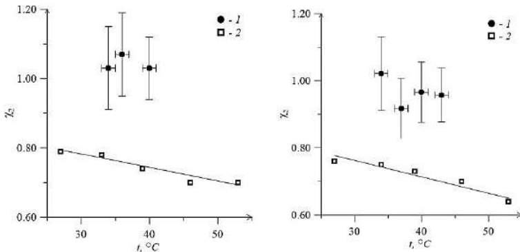
Рис. 3. Мнимая часть динамической восприимчивости в зависимости от температуры магнитной жидкости при частотах зондирующего поля 10 и 12 кГц соответственно. 1 – результаты измерений по тепловыделению, 2 – мостом взаимной индуктивности. Прямыми показана линейная аппроксимация результатов полученных на мосте
