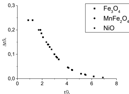
Рис. 4. Зависимость \Delta r(r/\lambda)/\lambda от r/\lambda для \text{Fe}_3\text{O}_4 , \text{MnFe}_2\text{O}_4 и \text{NiO} .
