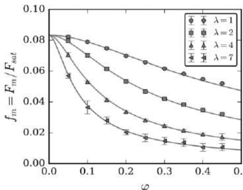
Рис. Нормированная магнитная сила, действующая на кластер, как функция объемной доли частиц в кластере. \xi_c = 0.25 . Символы – результаты моделирования для N = 500 и g = 0.001 . Различные символы соответствуют различным параметрам диполь-дипольного взаимодействия. Кривые построены с помощью уравнений (7) и (8) для тех же параметров.
